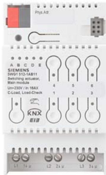
N 512/11 SWITCH ACTUATOR MAINMODUL 3X AC 230V, 16A
