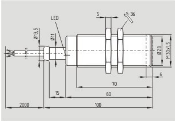
Maßzeichnung (Grundgerät)
