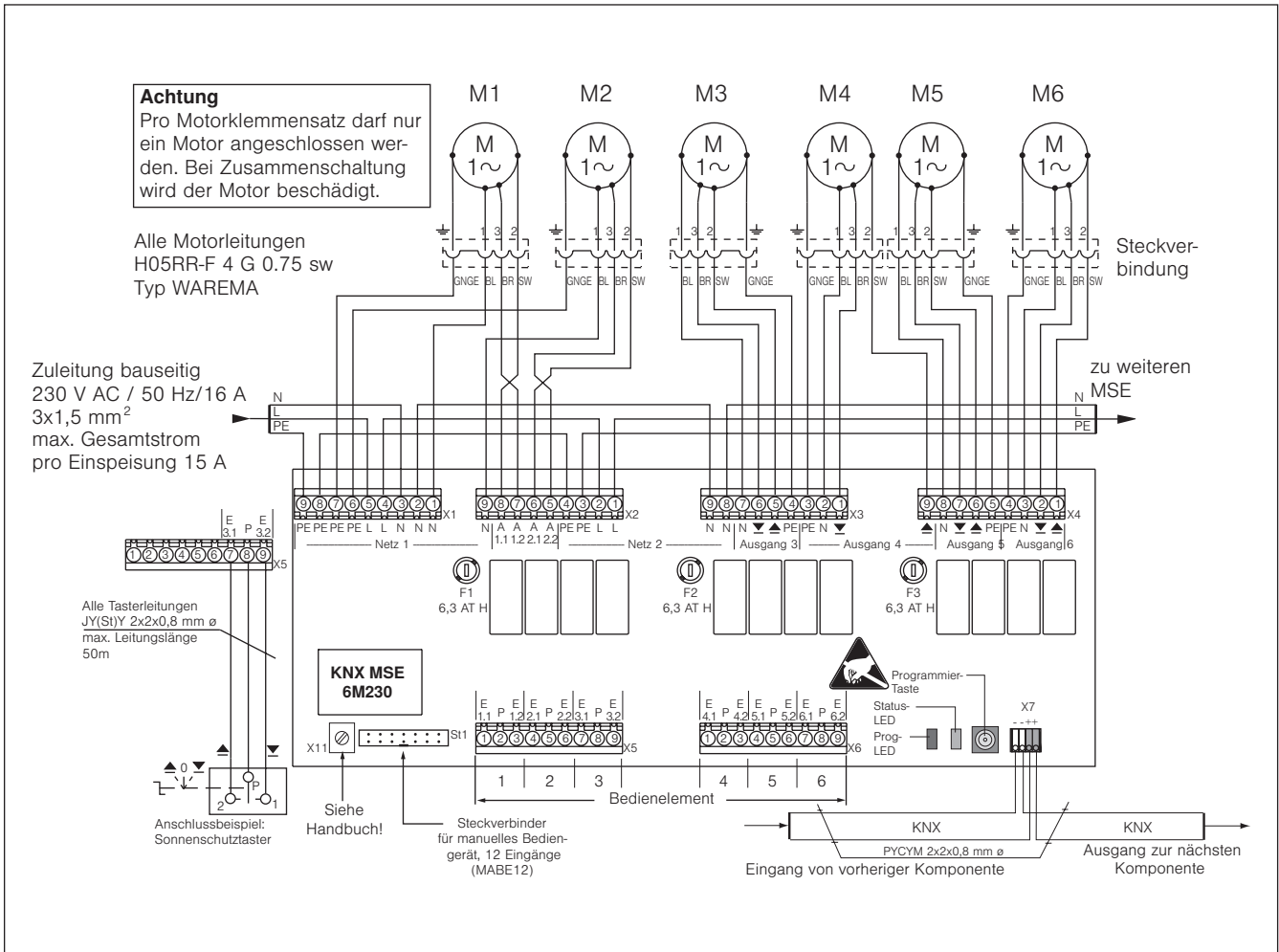
Abb. 6 KNX MSE 6M230 / 6 Antriebe
