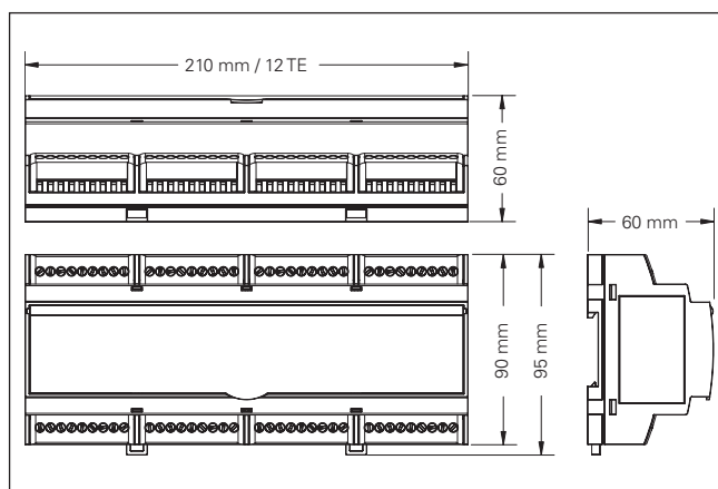
Abb. 5 Abmessungen Reiheneinbaugehäuse 12 TE
