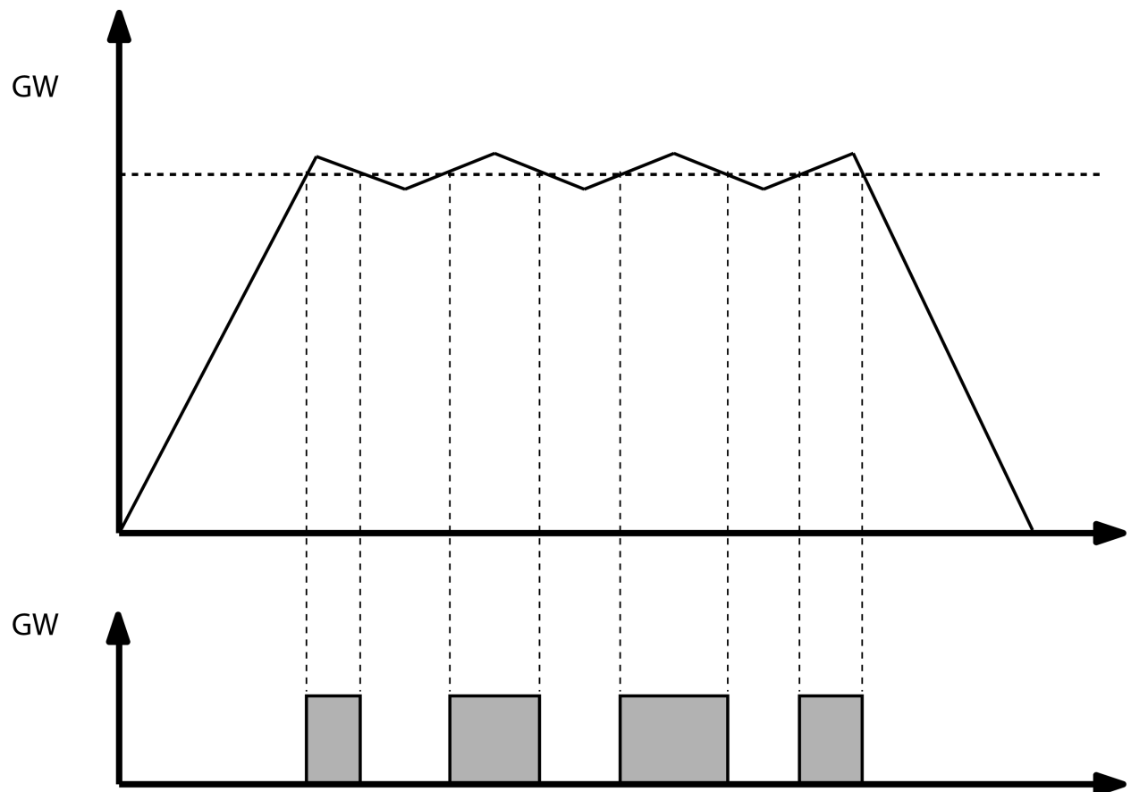
Bild 12: Schalthäufigkeit ohne Hysterese
