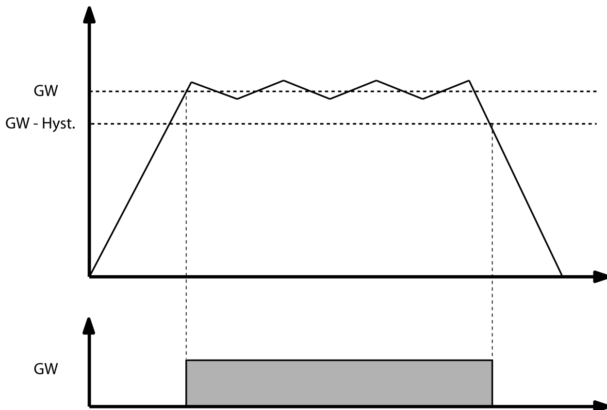
Bild 13: Schalthäufigkeit mit parametrierter Hysterese
