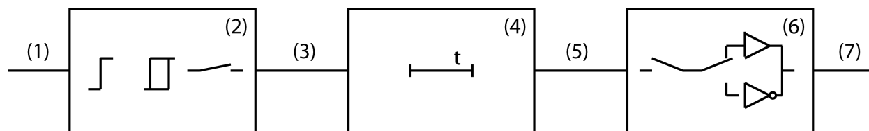
Bild 15: Blockdiagramm Ein- und Ausschaltverzögerung
