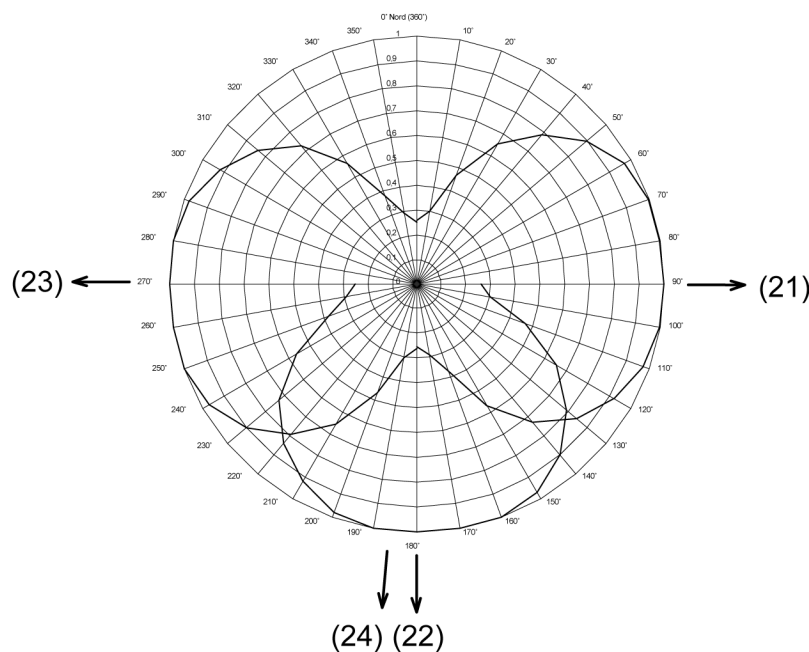
Bild 11: Kreisdiagramm Helligkeitserfassung
