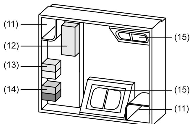
Bild 3: Unterteil Klemmenkasten (9)
