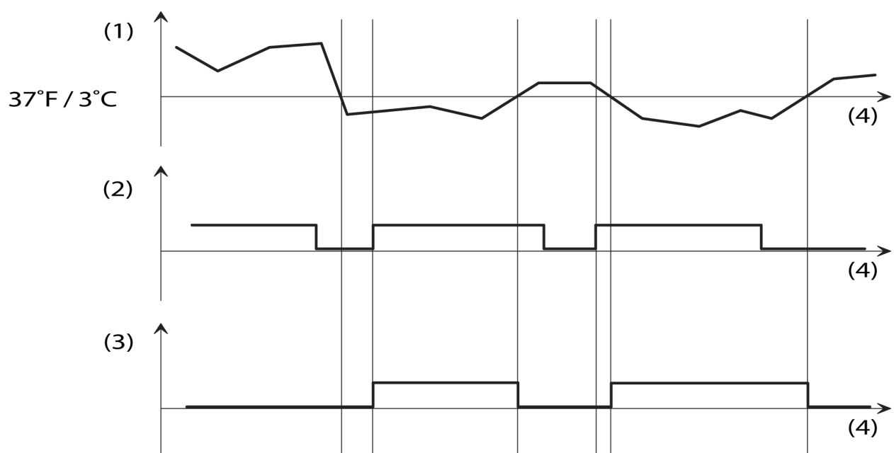
Bild 8: Vereisungsschutz in Abhängigkeit von Temperatur und Niederschlag
